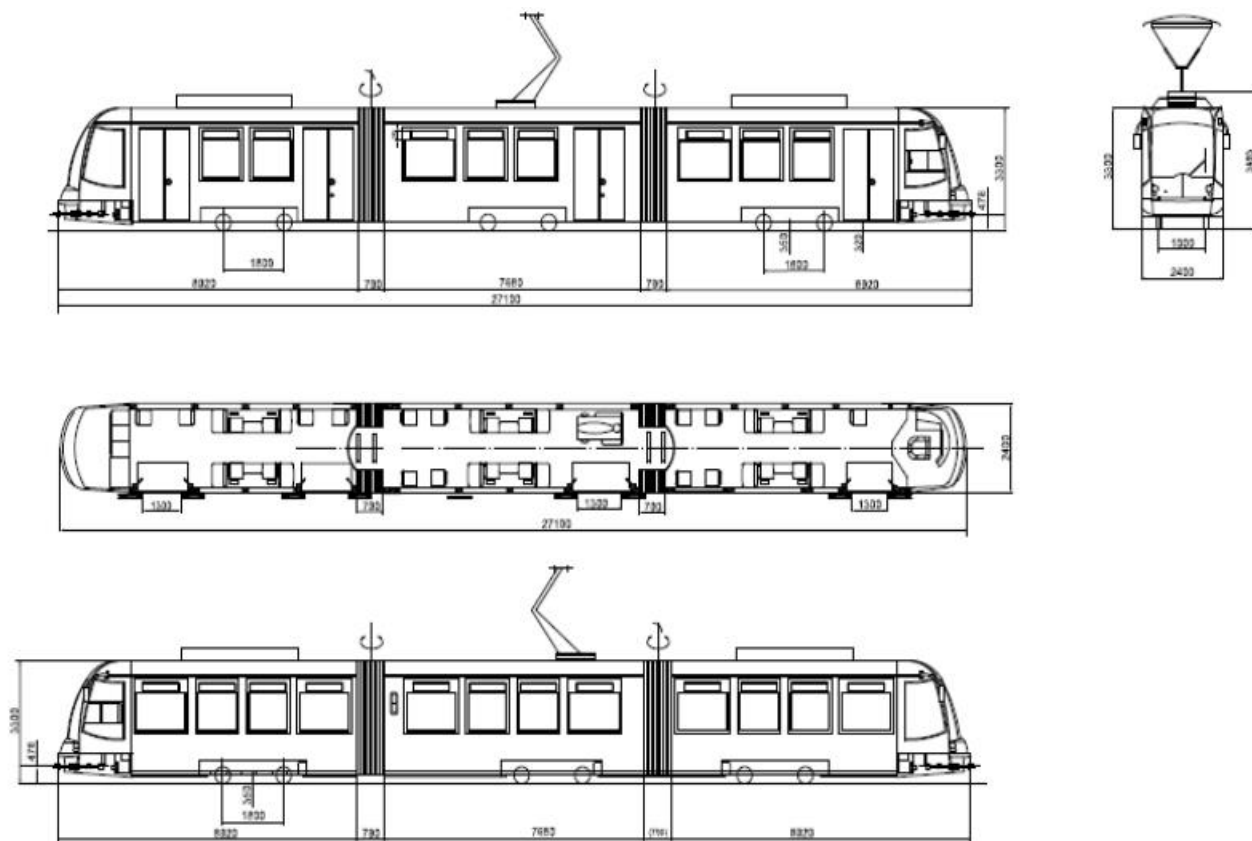
Fig.13. Tramvai Imperio
