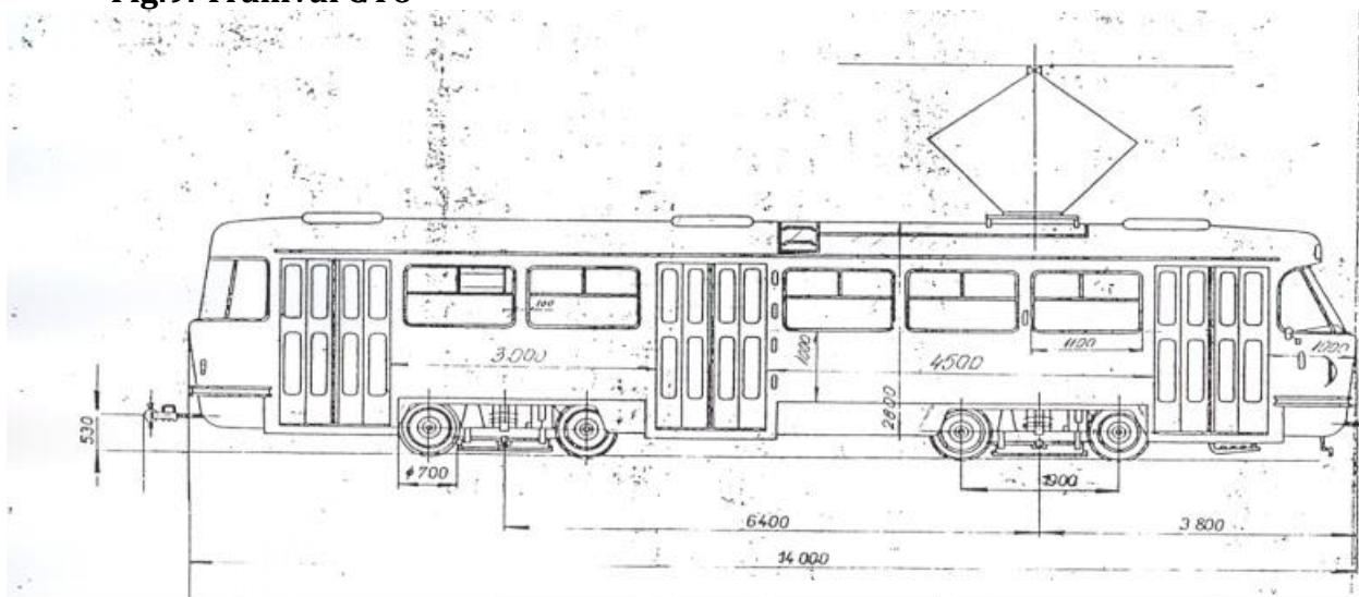
Fig.9. Tramvai GT6
