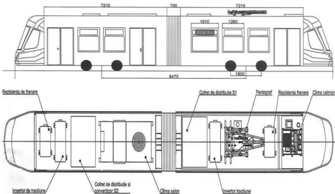
Fig.13. Tramvai Imperio
