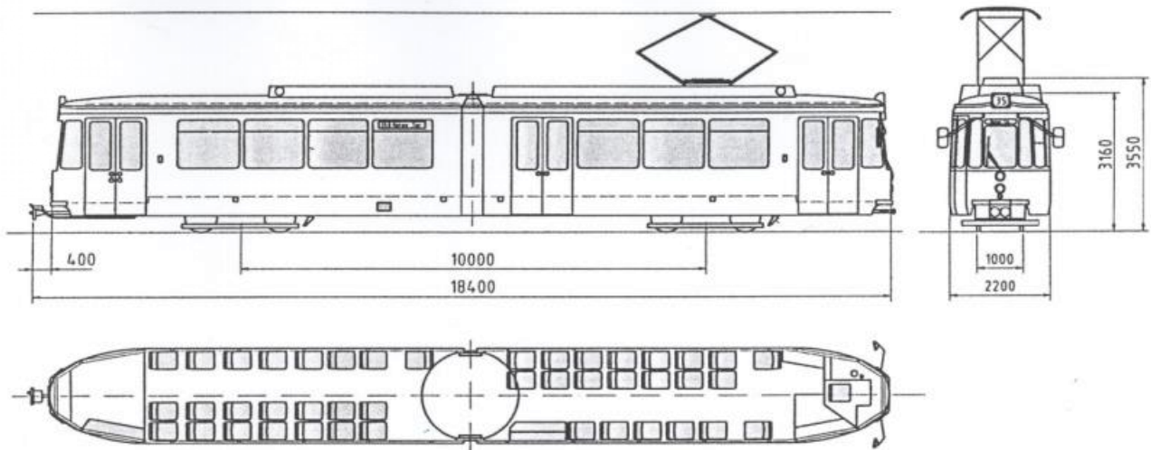
Fig.8. Tramvai GT4
