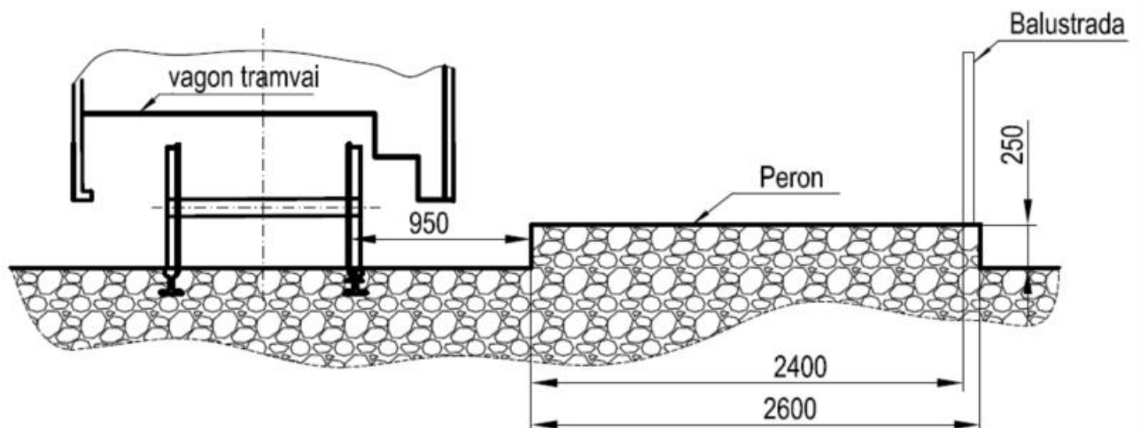
Fig.7. Secțiunea transversală în stația Primărie
