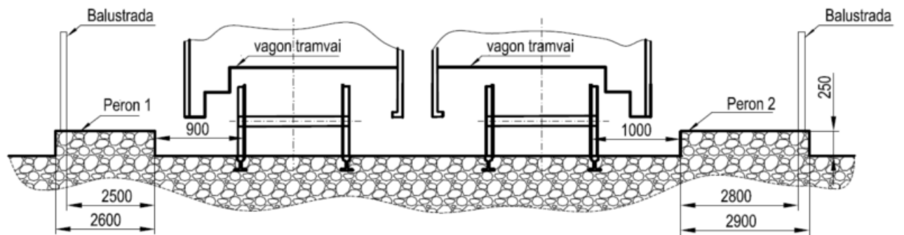
Fig.6. Secțiunea transversală în stația Gară
